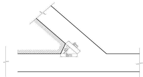
Kích thước vật góc tại góc cắt nhau nhau với lộ giới lớn hơn hoặc bằng 45^{\circ}
