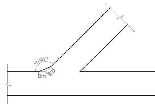
Kích thước vật góc tại góc cắt nhau nhau với lộ giới nhỏ hơn hoặc bằng 135^{\circ}
